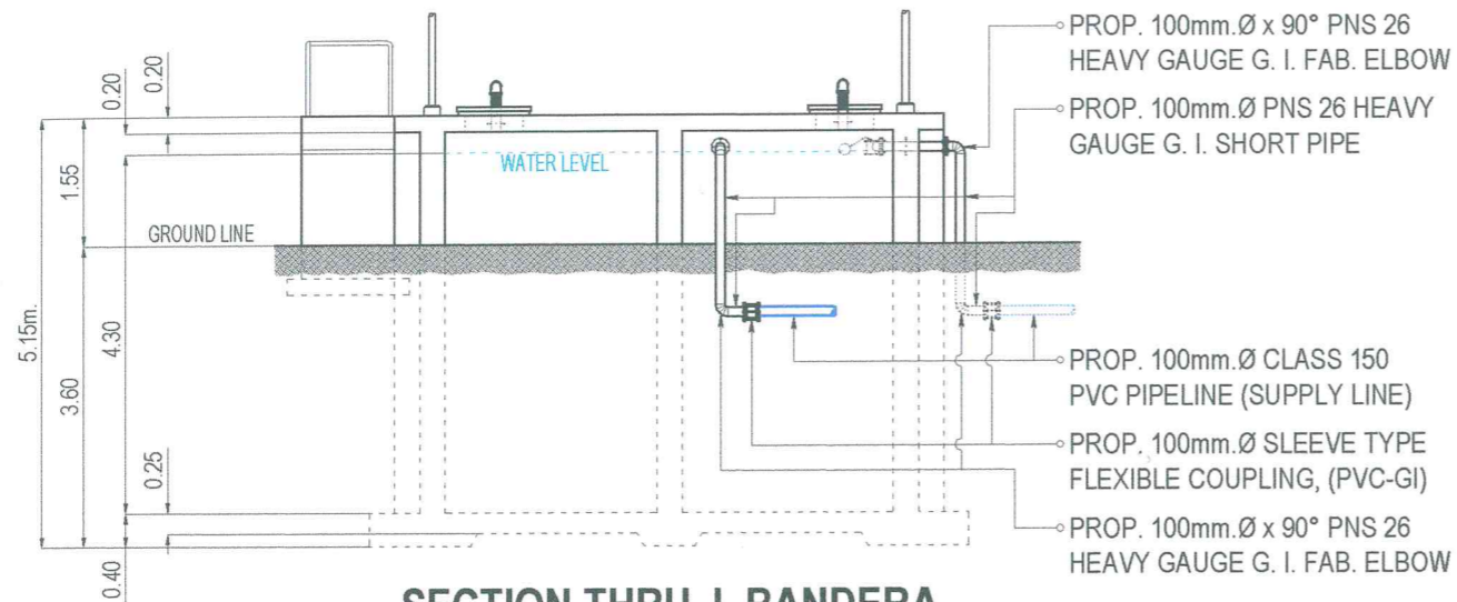
SECTION THRU J, BANDERA SCALE: 1:100 M.
