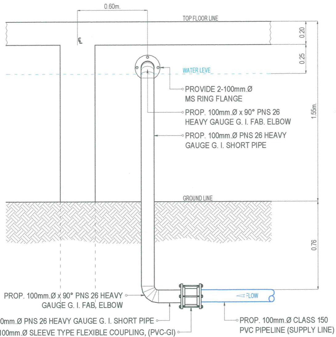
SECTION THRU J, BALUNO SCALE: 1:20 M.
